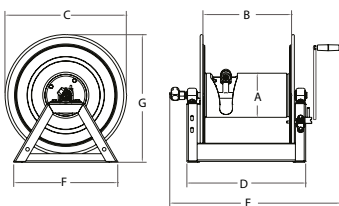
1185 SERIE MOTOR
