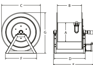
1195 SERIE MOTOR
