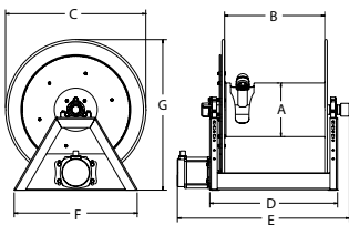
1195 SERIE MOTOR
